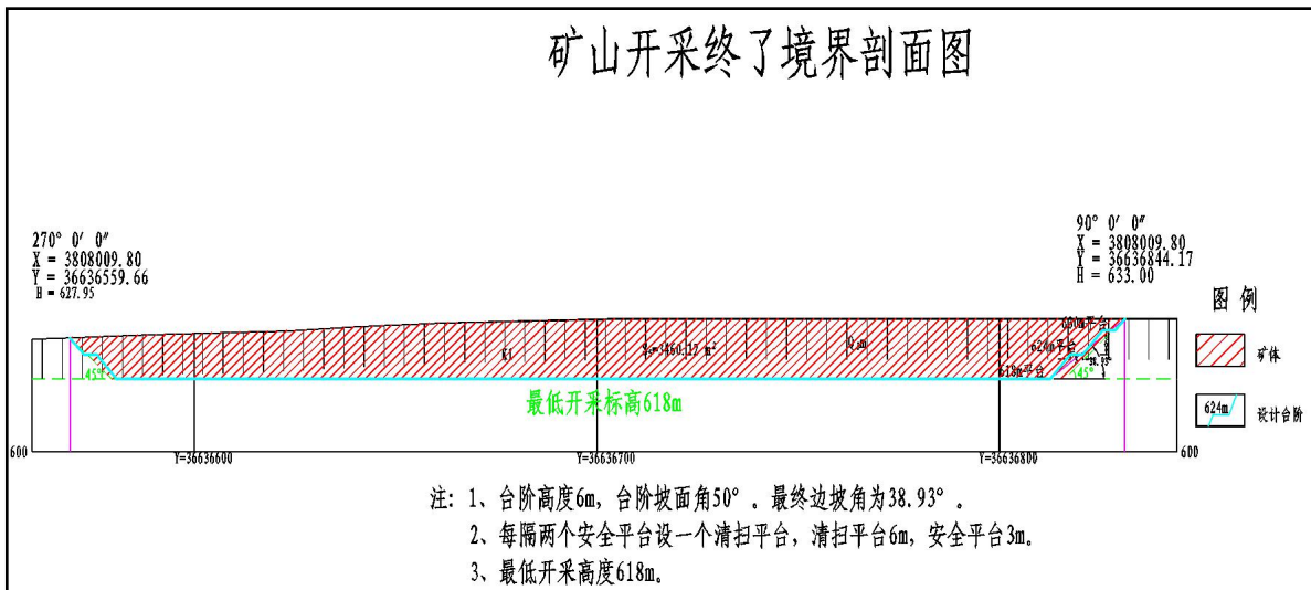
图 1.3-2 开采终了剖面图
