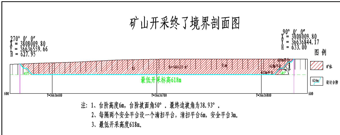
图 1.3-2 开采终了剖面图
