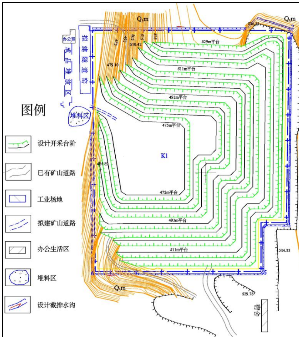
图 1.3-3 矿山工程平面布置示意图
