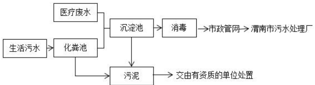
图 4-1 污水处理工艺流程
