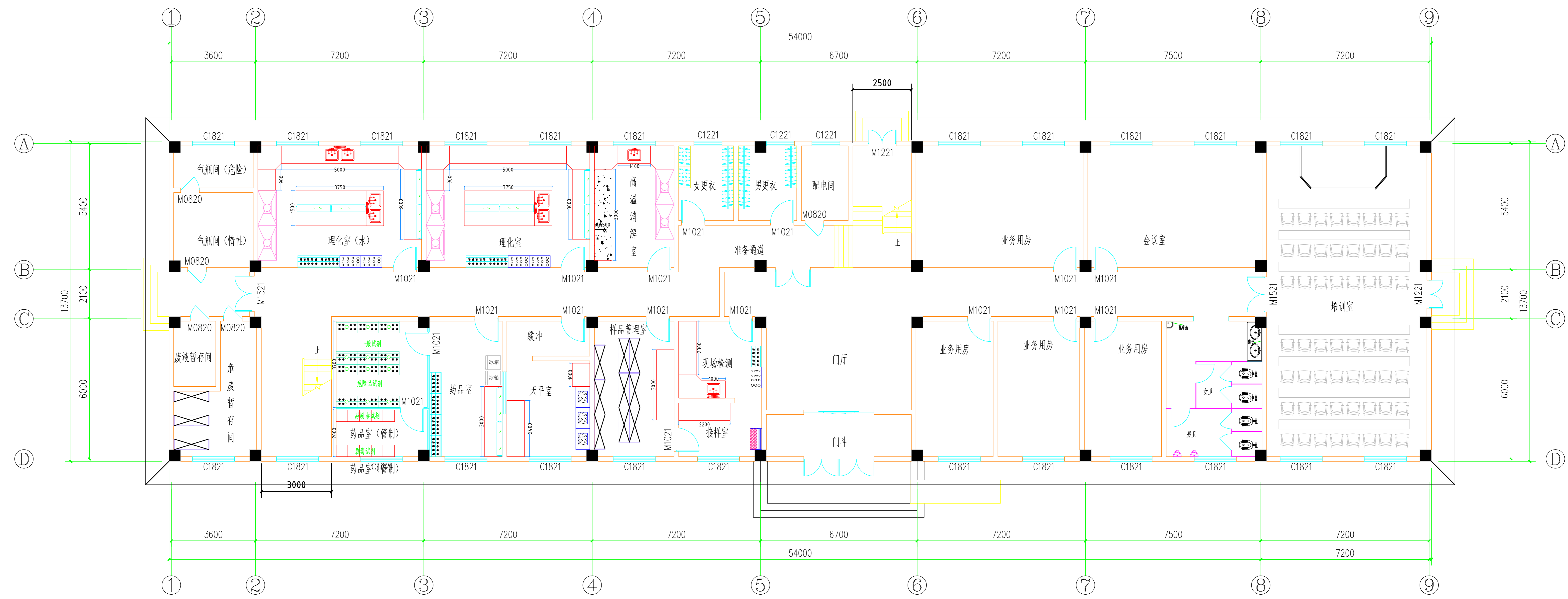
一层平面图 1:100 单层面积: 729.00m 2 整栋楼为一个防火区
