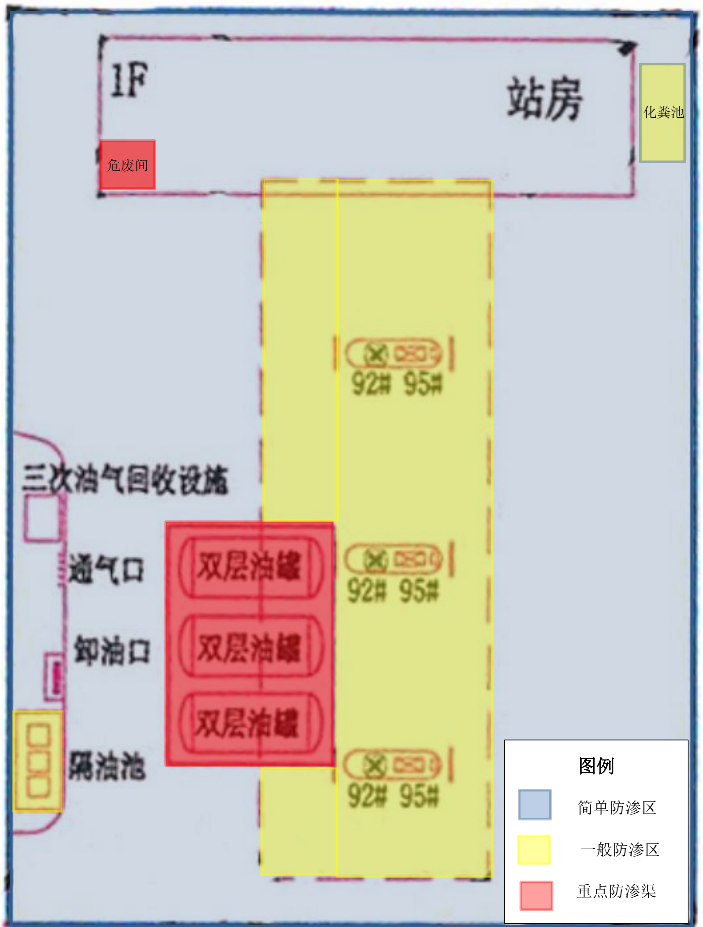
附图 7 项目分区防渗图
