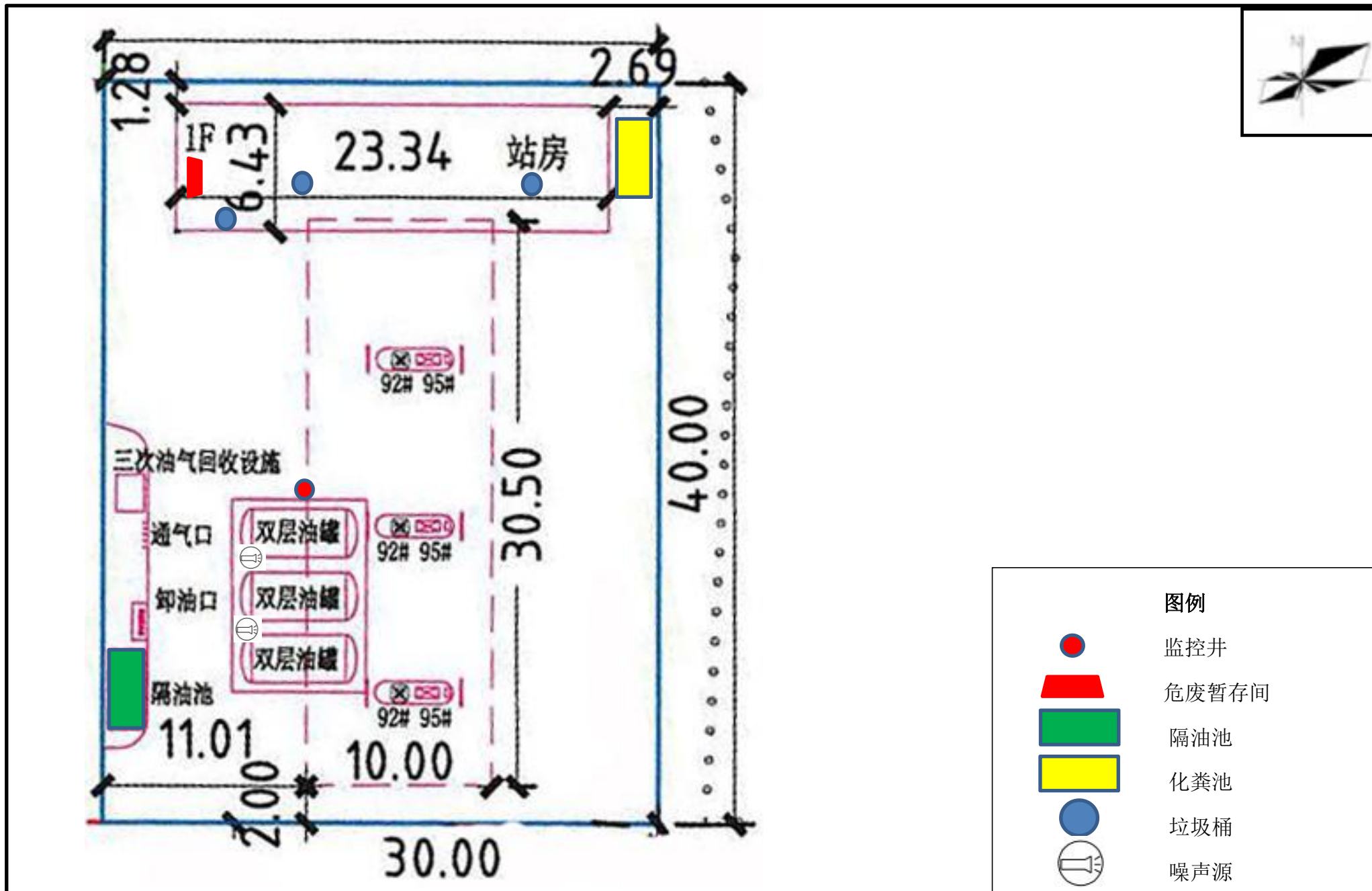
附图2 项目平面布置图 (单位: m)
