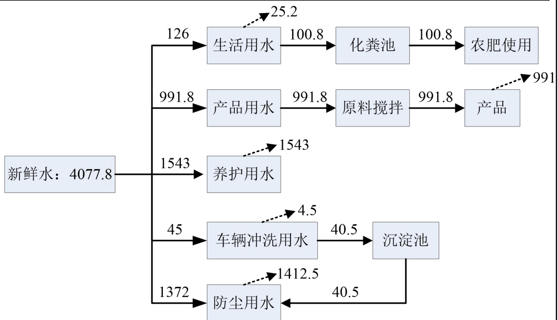
图 1 全厂水平衡图 单位 m 3 /a
