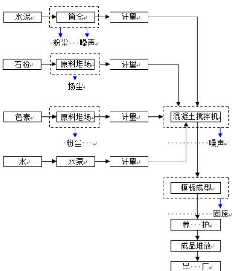
图3 水泥预制件生产工艺流程及产污环节示意图
