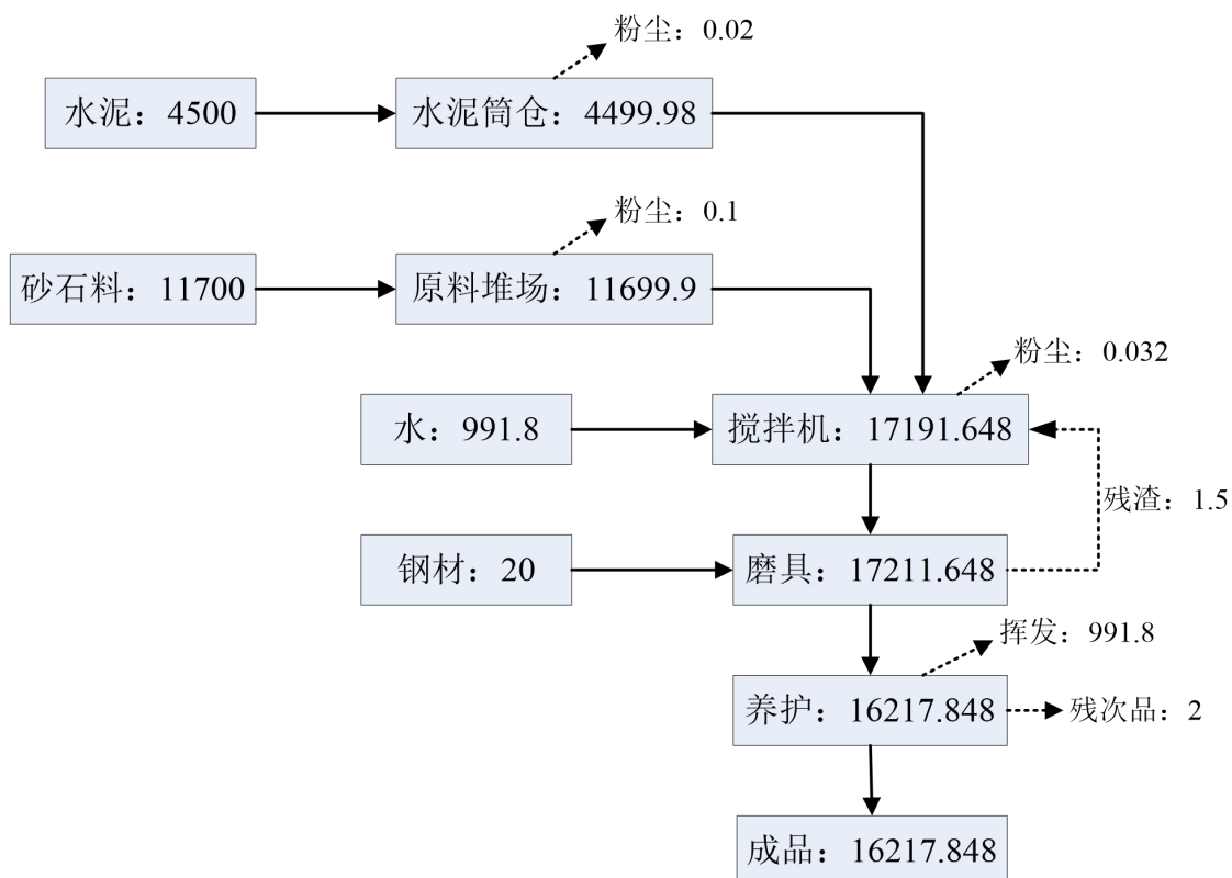
图 4 项目生产过程物料平衡图 单位: t/a
