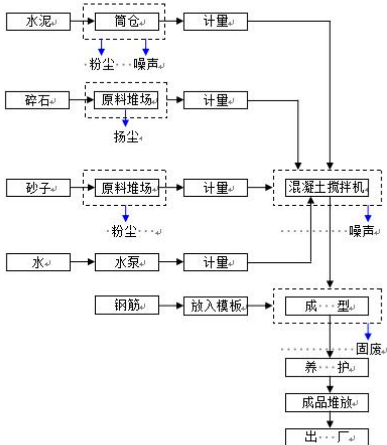
图2 水泥混凝土制品生产工艺及产污环节示意图
